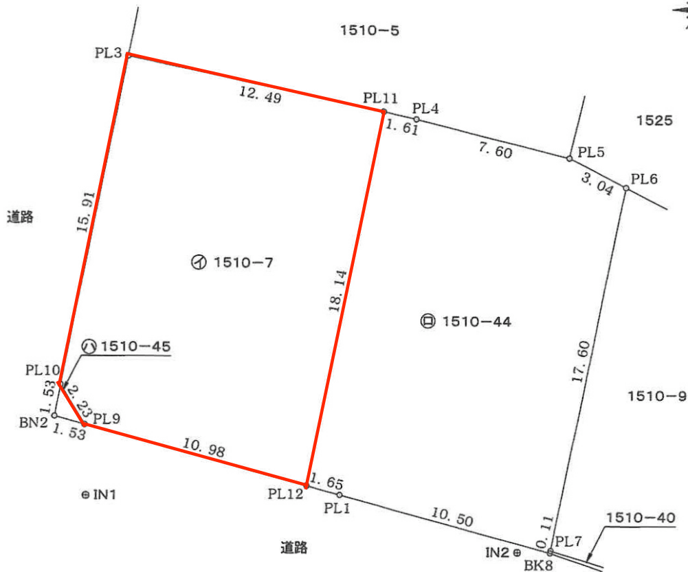
引照点詳細図
